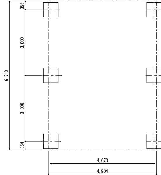
■基礎配置図
